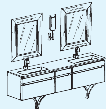
COMPOSIZIONE 10 cm L 70 P 52 H 200
