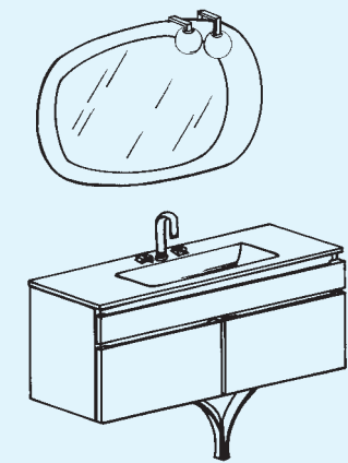
COMPOSIZIONE 4 cm L 110 P 52 H 190
